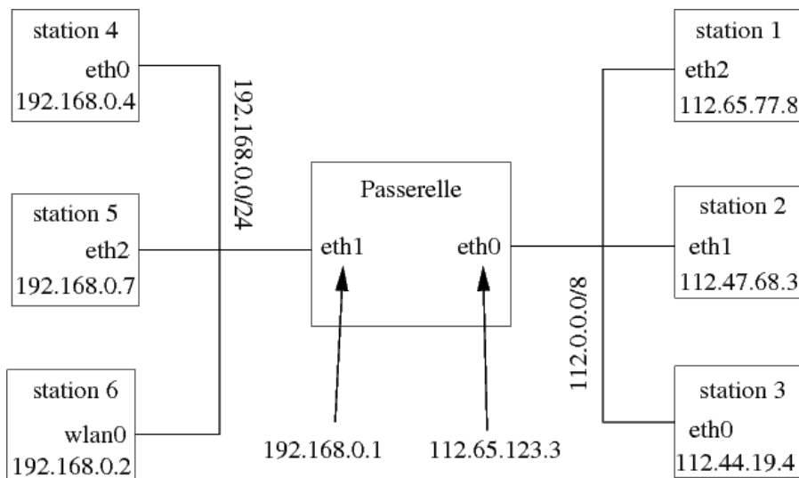
FIGURE 8.1: Exemple de passerelle faisant communiquer deux réseaux
