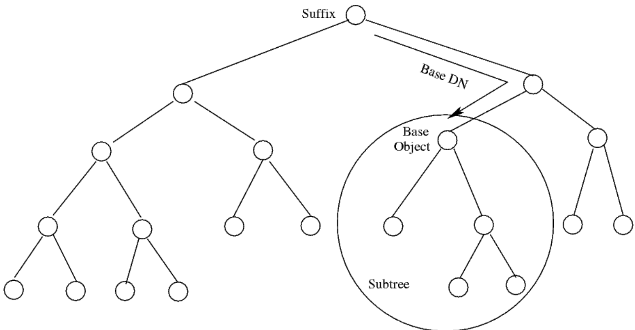
FIGURE 11.3: Le base object et le subtree d'une requête.
